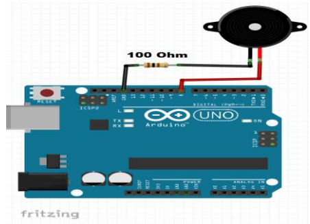
Fig.10. Buzzer with Arduino UNO
